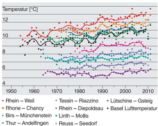
Abb. 10: Wassertemperaturverlauf der letzten Dekaden für neun ausgewählte Stationen und Basel (Lufttemperatur). Für Stationen mit kalten mittleren Wassertemperaturen (z. B. Lüttschine-Gsteig) ist der Temperatur-sprung zwischen 1987 und 1988 weniger deutlich als z. B. im Ticino. Zudem fällt die geringere Schwankung der Lüttschine-Wassertemperatur innerhalb eines Jahres auf (interannuelle Variabilität). Beides veranschaulicht den ausgleichenden Effekt der Gletscher. Quelle: BAFU.
