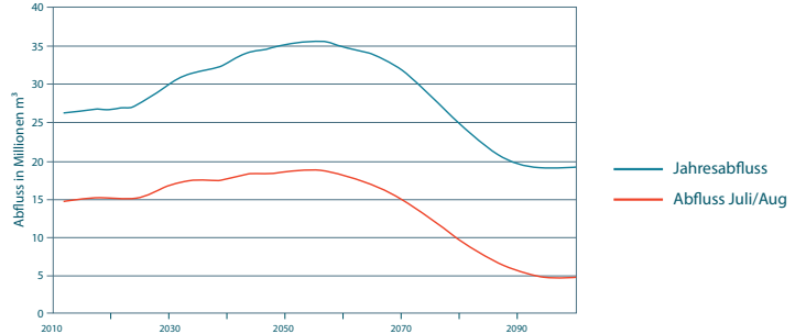
Abb. 5: Zukünftiger Verlauf der Abflüsse vom Plaine-Morte-Gletscher.
