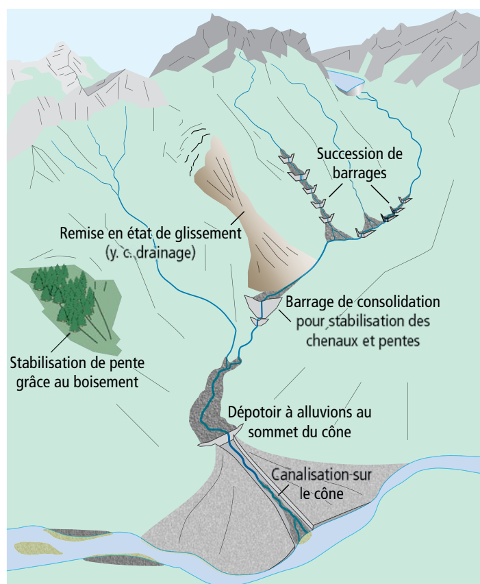
Fig. 55: Différents types de mesures préventives dans les bassins versants des torrents. 100
