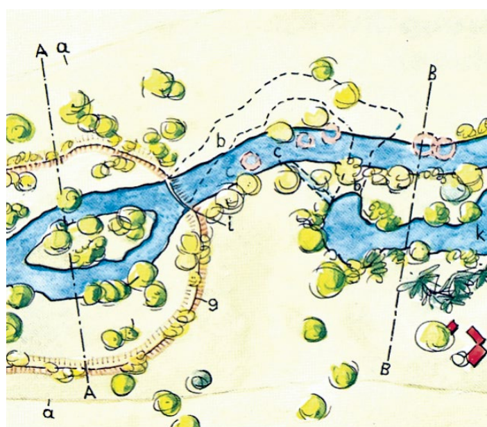
Fig. 63 : La représentation du système étroit avec digues et barrières (Sporensystem), utilisé notamment sur le Rhône au XIX e siècle (à gauche) et celle du concept « Davantage d'espace pour les cours d'eau », issu de la directive « Protection contre les crues des cours d'eau » de 1982 (à droite), montrent clairement le changement intervenu dans la protection contre les crues entre le XIX e siècle et aujourd'hui.
