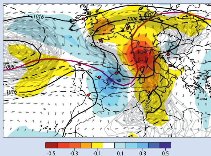
Fig. 44: Pression au sol réduite (hPa; lignes noires continues; lignes grises pour l'ensemble), vent à 850 hPa (1,5 km d'altitude; flèches grises), pression à 500 hPa (env. 5 km d'altitude; lignes noires pointillées), mouvement vertical des masses d'air à 500 hPa (les valeurs négatives signifient un mouvement ascendant) et tropopause (1,5 PVU; ligne rouge), tiré de 20CR pour le 22 septembre 1868 à 12 UTC. Les endroits des mesures utilisées pour établir 20CR sont indiqués par des points rouges.
