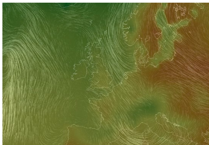
Fig. 43: Température au sol et lignes de courant le 14 juin 1910 à 12 UTC dans la réanalyse CERA-20C.
