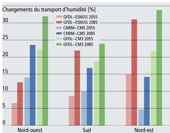
Fig. 11 : Changements (en pourcents) de l'intensité des épisodes extrêmes de transport d'humidité pour le nord-est de la Suisse, le nord-ouest de la Suisse et le sud des Alpes, tels que calculés par trois modèles climatiques globaux différents. Les couleurs claires montrent les changements d'ici à la moitié du 21 ème siècle, les couleurs foncées d'ici à la fin du 21 ème siècle. Les trois modèles montrent une augmentation claire de l'intensité des épisodes extrêmes de transport d'humidité.
