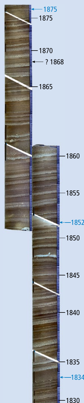
Fig. 67: Dépôts de crue dans le lac d'Oeschinen de 1830 à 1875. 128
