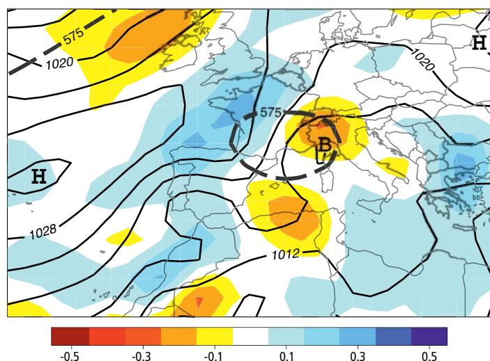
Fig. 8 : Situation météo pendant l'inondation le 21 août 2005. 25 En dessous d'une goutte froide à 500 hPa (env. 5 km d'altitude, en gras 12 ), une dépression de Gênes se développe (« B », des lignes continues montrent la pression au sol en hPa) qui est bloquée entre deux hautes pressions (« H »). Les couleurs montrent les vents verticaux à 500 hPa (Pa/s, couleurs rouges pour les vents ascendants).
