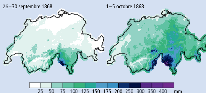
Fig. 48: Accumulations de précipitation sur 5 jours au Tessin telles que reconstruites par la méthode des analogues sur une grille de 2 km et pour les périodes suivantes: 26–30 septembre et 1–5 octobre 1868.
