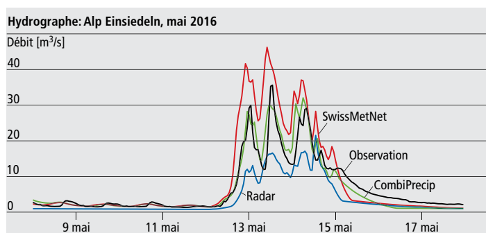
Fig. 37: Simulation de débit de la rivière Alp près d'Einsiedeln [ m^3 s^{-1} ] avec le modèle hydrologique PREVAH pour la période du 8 au 17 mai 2016. Trois données de précipitations ont été utilisées pour les simulations : données SwissMetNet interpolées (rouge), données radar (bleu) et le produit CombiPrecip (vert).
