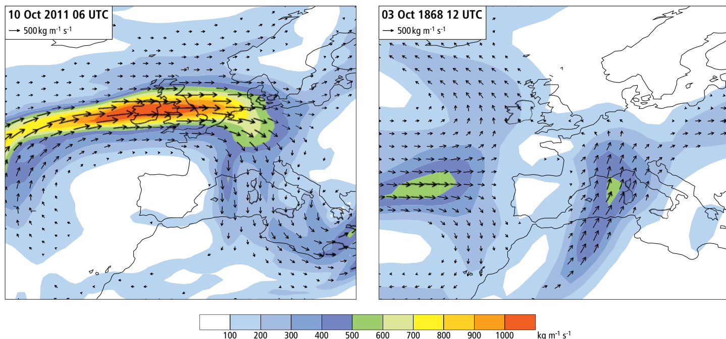
Fig. 10: Transport d'humidité atmosphérique intégré verticalement ( \text{kg m}^{-1} \text{s}^{-1} , en couleurs) pour le 10 octobre 2011 à 6 UTC (gauche) et le 3 octobre 1868 à 12 UTC (droite). Les flèches montrent la direction du transport. La rivière atmosphérique est reconnaissable à gauche par une longue structure allongée. L'air humide a atteint les Alpes par le nord le 10 octobre 2011 et par le sud le 3 octobre 1868. 25
