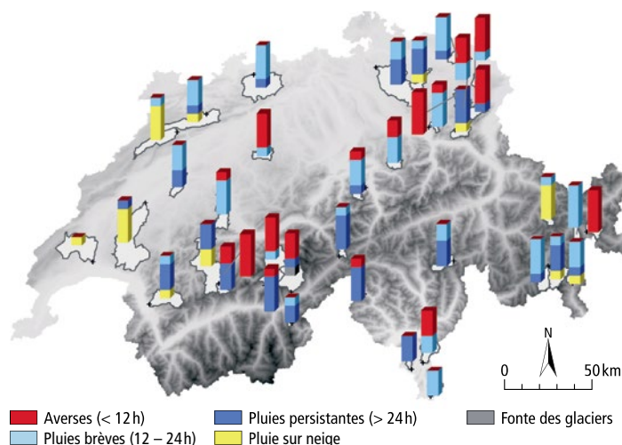
crue élevées et des inondations dues à de trop hauts niveaux de lacs Fig. 23 : Fréquence pondérée des types de précipitations déclencheuses dans quelques bassins versants choisis. La pondération donne une plus grande importance à un type de précipitation qui provoque une grande crue qu'à un type qui ne génère qu'une petite crue.
