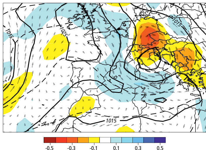
Fig. 42: Carte météorologique tirée de la ré-analyse 20CR 25 pour le 14 juin 1910 à midi (12 UTC): pression au sol réduite au niveau de la mer (hPa; lignes noires épaisses), champ de vent à 850 hPa (env. 1,5 km d'altitude; flèches grises), pression à 500 hPa (env. 5 km d'altitude; lignes pointillées épaisses), mouvement vertical des masses d'air à 500 hPa (les valeurs négatives signifient un mouvement ascendant).
