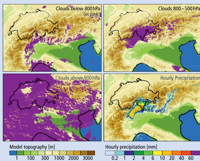
Fig. 47: Couverture nuageuse et précipitation horaire (en bas à droite) dans le modèle WRF sur une grille de 2 km pour le dimanche 27 septembre 1868 à 3 h. La couverture nuageuse en violet correspond aux basses couches (en haut à gauche), couches moyennes (en haut à droite) et hautes couches (en bas à gauche).
