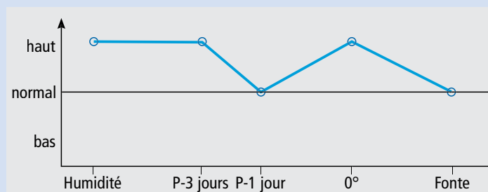
Fig. 26: Représentation schématique de l'impact des facteurs variables sur l'événement de crue de 1868 (voir fig. 22 pour les facteurs).
