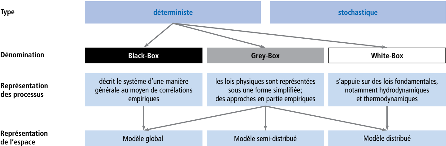
Fig. 49: Résumé des différents types de modèles en hydrologie. Pour la reconstruction d'événements de crue, les modèles grey-box constituent souvent le bon choix. 70
