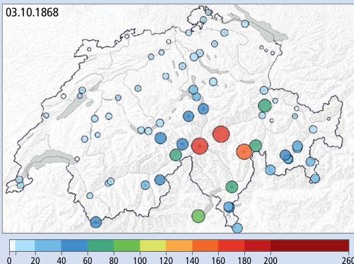
Fig. 33: Mesures de la quantité de précipitations journalière (mm ou litres par m 2 en 24 heures) en Suisse le 3 octobre 1868. 12,32
