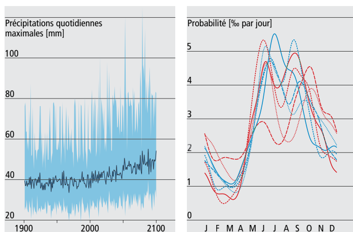
Fig. 75: (à gauche) Évolution des précipitations journalières maximales par année pour le bassin versant de l'Aar, tirée des simulations CMIP5 (bleu foncé : valeur moyenne de toutes les simulations, bleu clair : maxima et minima). (à droite) Jour calendaire des précipitations journalières maximales d'une année dans le passé (bleu, 1971–2005) et le futur (rouge, 2065–2099, différentes cotes en pointillés représentent différents ensembles de modèles). 148
