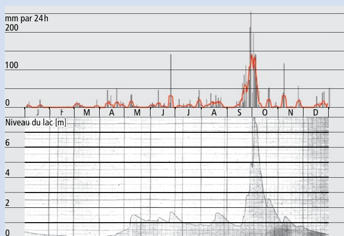
Fig. 34: (en haut) Accumulations journalières (barres noires) et accumulations sur cinq jours (ligne rouge) des précipitations à la station San Bernardino Ospizio à l'altitude du col. (en bas) Le niveau du lac Majeur à Verbania en 1868. 48
