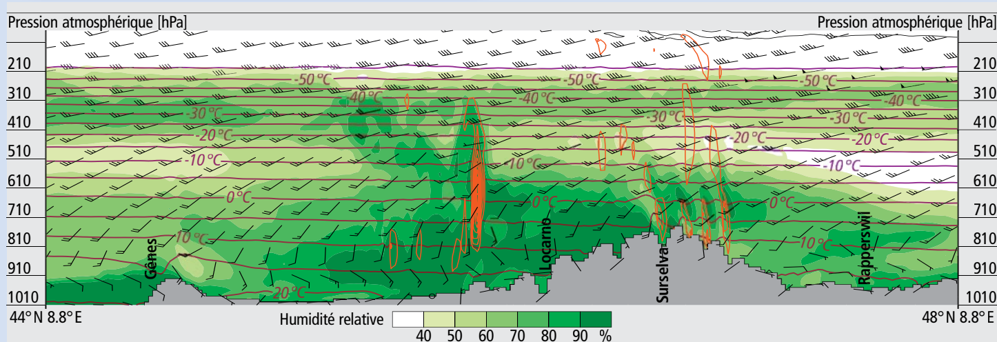
Fig. 16: Coupe verticale sud-nord (sud à gauche, nord à droite) au-dessus des Alpes pour le 26 septembre 1868 à 21 UTC. Les données proviennent d'une simulation avec le modèle météo WRF (cf p. 26) sur une grille de 2 km de côté et comprenant 40 couches. La topographie en gris foncé correspond à la topographie du modèle. Les couleurs montrent l'humidité relative. Le vent horizontal est représenté par des flèches à barbules: pointant vers le haut pour un vent du sud (vent venant du sud) pointant à droite pour un vent d'ouest, etc. Plus les flèches contiennent de barbules (traits obliques), plus il y a de vent (10 nœuds, soit environ 20 km/h pour un barbule). Les contours rouges indiquent les courants ascendants. La température est montrée par des lignes noires. La limite du 0 degré se situe aux alentours de 630 hPa (environ 4 km au-dessus de la mer).
