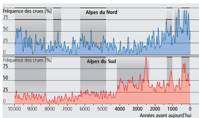
Fig. 66: Fréquence des crues dans les Alpes du Nord (10 lacs) et les Alpes du Sud (5 lacs) au cours des 10 000 dernières années. 130
