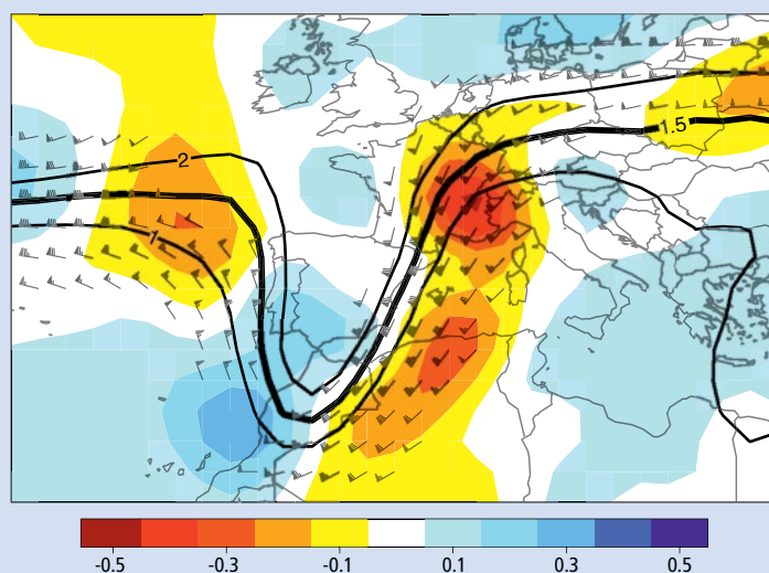
Fig. 9 : Situation météo avec PV-streamer le 3 octobre 1868 à midi. 25 Des lignes continues montrent les unités de PV (1.5 PVU en gras pour la tropopause). Les flèches avec barbules indiquent la bande de forts vents dans la haute troposphère (à 250 hPa, seules les vitesses de plus de 50 nœuds sont montrées). Les couleurs montrent les vents verticaux (Pa/s, couleurs rouges pour les vents ascendants) dans la moyenne troposphère (500 hPa).
