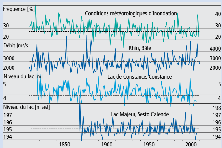
Fig. 73: Débit annuel maximum du Rhin à Bâle, ainsi que niveau maximal du lac de Constance et du lac Majeur. 32 La ligne du haut montre la fréquence des conditions météorologiques «septentrionales cycloniques» et «occidentales cycloniques» sur le sud de l'Europe (mai à octobre), typiques pour les crues sur le versant nord des Alpes (en pointillé: moyennes 1951–2000).
