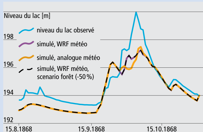
Fig. 50: Reconstruction de précipitations et de saturation du sol (valeurs moyennes régionales, à gauche), ainsi que du niveau du lac (à droite). Les barres bleues à droite dirigées vers le haut montrent les précipitations de l'affinage numérique par la simulation WRF (sur fond gris). Les barres bleues dirigées vers le bas et les barres situées à l'extérieur de la surface grise proviennent de la méthode des analogues (affinage statistique) (cf p. 27)
