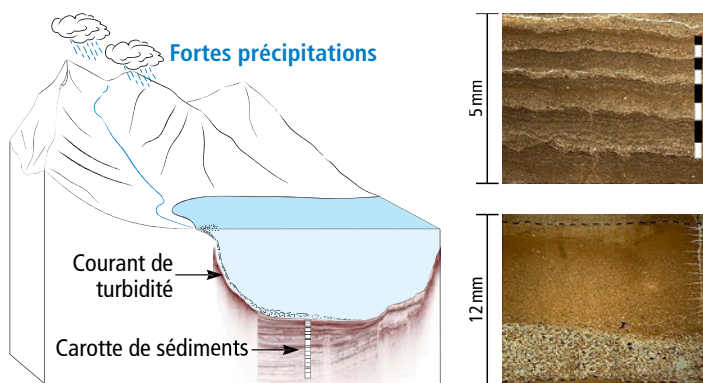
Fig. 64 : Schéma d'un bassin versant avec la sédimentation d'un dépôt de crue et la position d'une carotte de sédiments (diagramme de gauche). 129 A droite, es sédiments du lac d'Oeschinen 1 montrent (en haut) une sédimentation normale, calme, avec quatre dépôts annuels (la couche claire représente chaque fois le printemps avec la fonte des neiges) et (en bas) un dépôt de crue de 12 mm avec des grains de sable grossiers à la base et une fine couverture limon/argile. 128
