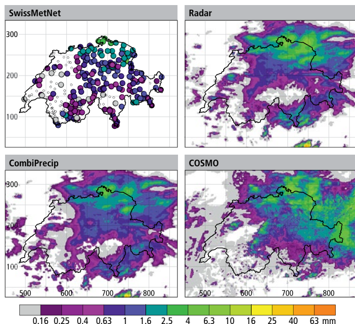
Fig. 36: Quantité de précipitations [mm] tombée entre 11 et 12 UTC le 12 mai 2016 telle que mesurée par les stations du SwissMetNet (en haut à gauche), évaluée à l'aide du radar (en haut à droite), évaluée à partir de la combinaison de données des stations et des radars (CombiPrecip, en bas à gauche) et dans l'analyse du modèle de prévision météo COSMO.
