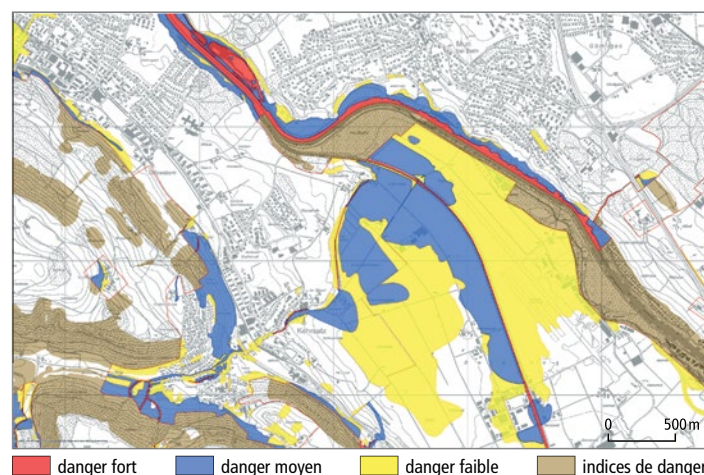
Fig. 3: Détail de la carte des dangers naturels du canton de Berne, région de Kehrsatz-Belpmoos.
