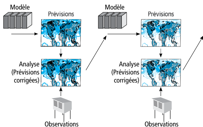
Fig. 39 : Déroulement schématique d'une réanalyse.
