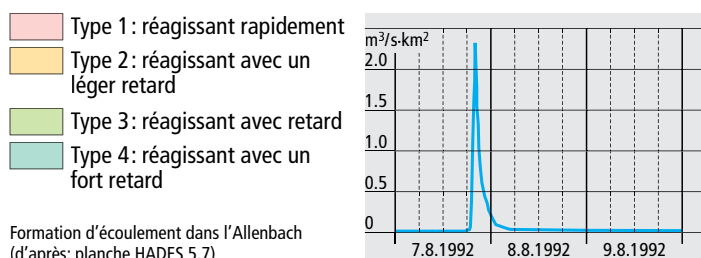
Fig. 17: Formation d'écoulement dans l'Allenbach à Adelboden: 1 évaluation de la prédiposition de fond. 36
