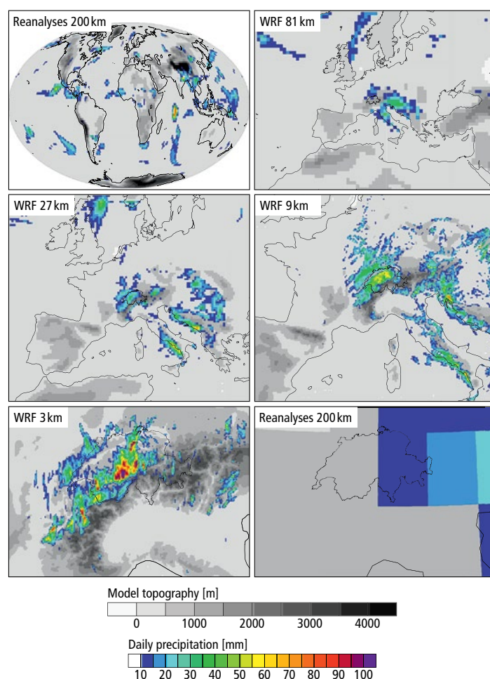
Fig. 45: À partir de la réanalyse 20CR, des simulations WRF sont effectuées sur une grille de 81, 27, 9 et finalement 3 km de côté. Les précipitations journalières simulées pour le 22 août 2005 sont montrées. La réanalyse est aussi montrée en bas à droite pour le même domaine que la simulation WRF à 3 km, pour comparaison.
