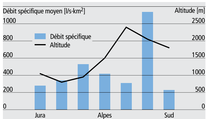
Fig. 18: Apport de débit [l/s·km²] d'une crue moyenne le long d'un profil nord-sud à travers la Suisse. 37
