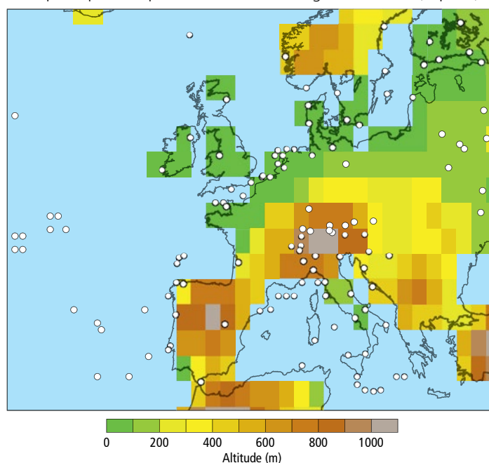
Fig. 41 : Mesures de pression pour la réanalyse 20CR 25 du 14 juin 1910, 6–12 UTC.
