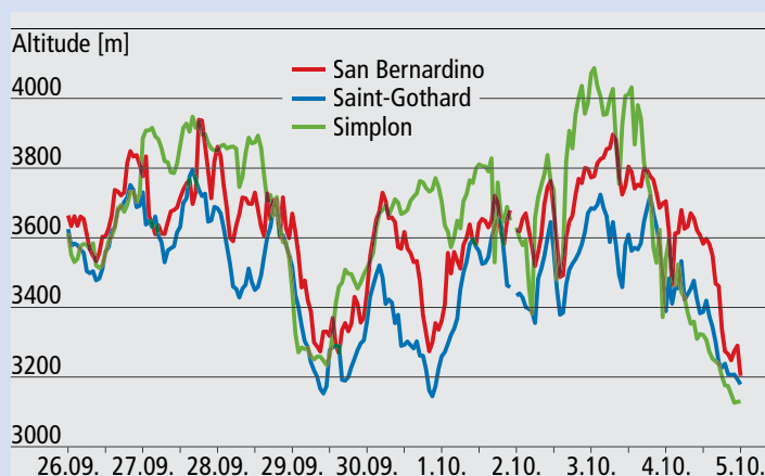
Fig. 25: La limite du zéro degré sur trois sites choisis, 1 reconstituée à l'aide d'un modèle météo régional (cf p. 26), montre que cette limite était à haute altitude de fin septembre à début octobre 1868. 32
