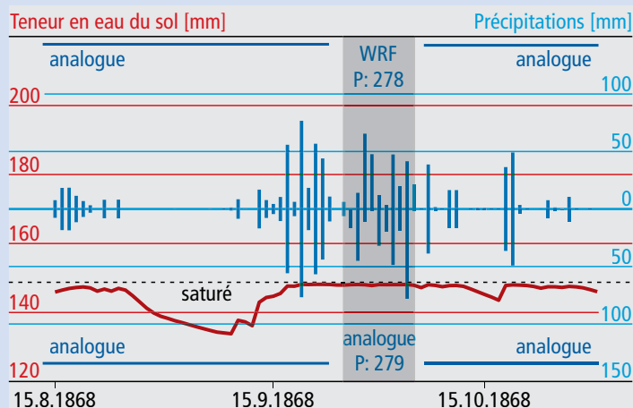
Fig. 50: Reconstruction de précipitations et de saturation du sol (valeurs moyennes régionales, à gauche), ainsi que du niveau du lac (à droite). Les barres bleues à droite dirigées vers le haut montrent les précipitations de l'affinage numérique par la simulation WRF (sur fond gris). Les barres bleues dirigées vers le bas et les barres situées à l'extérieur de la surface grise proviennent de la méthode des analogues (affinage statistique) (cf p. 27)
