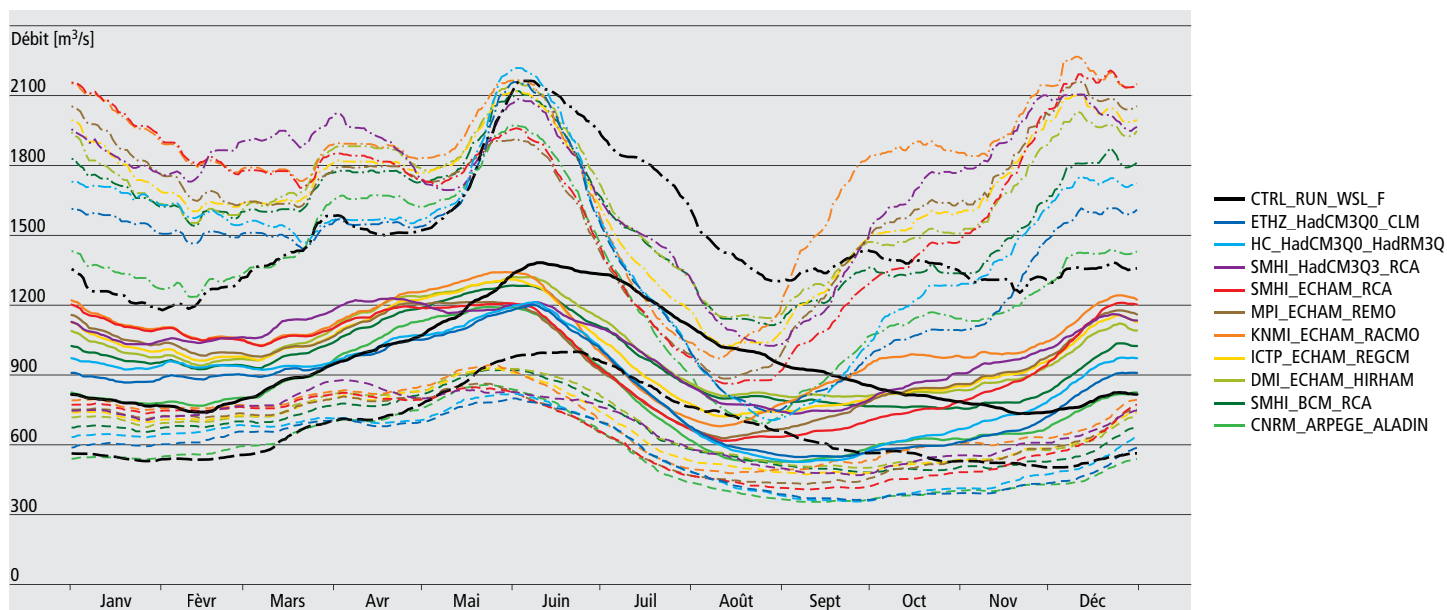
Fig. 76: Modification du débit du Rhin à Bâle. Représentation du quantile 10 % (pointillé), 50 % (continu) et 90 % (point-trait) pour la période de contrôle (1980–2010, noir) et pour dix scénarios climatiques (diverses couleurs) vers 2085. 149
