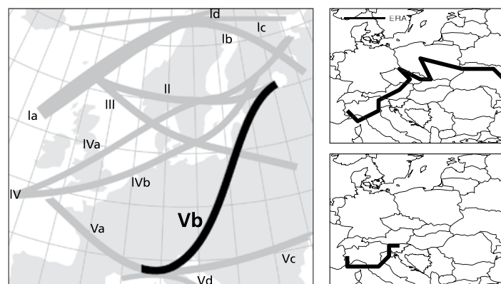
Fig. 6: Gauche : classification et dénomination des trajectoires des minima barométriques (basses pressions) par W.J. van Bebber. 16 Droite : trajectoires des dépressions pendant les inondations du 10 au 13 août 2002 (en haut) et du 20 au 24 août 2005 (en bas). 17,18
