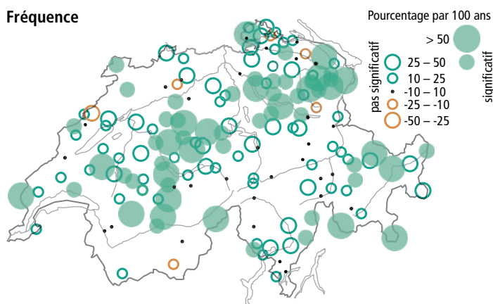
Fig. 70: Tendence (en % par siècle) de l'intensité des fortes précipitations (en haut; précipitations journalières maximales annuelles) et de leur fréquence (en bas, nombre de jours par année au-dessus du percentile 99 de tous les jours) aux stations de MétéoSuisse, 1901–2014. 139
