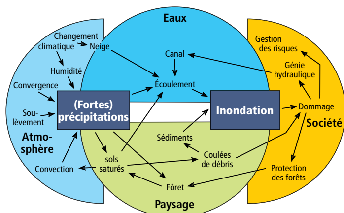
Fig. 2: Les fortes précipitations et les crues dépendent, de diverses manières, de processus météorologiques, hydrologiques, géomorphologiques et sociétaux.
