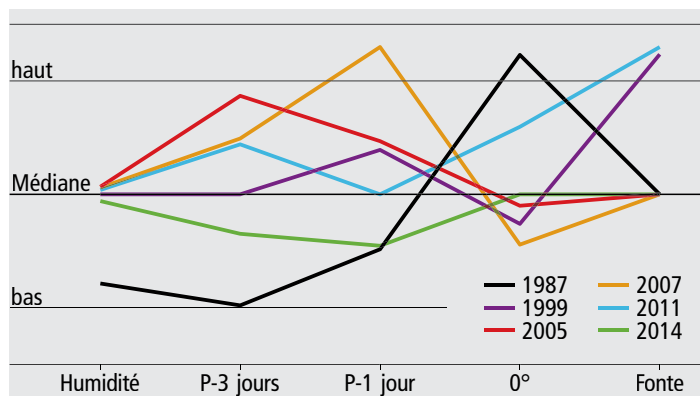
Fig. 22 : Prédiction variable et déclenchement des plus grandes crues de la Kander (cf fig. 21). Humidité : saturation du sol au début de l'événement ; jours P-3, jour P-1 : quantité de précipitations en 3 et 1 jour(s) ; 0° : altitude de la limite du zéro degré ; fonte : contribution de la fonte des neiges.
