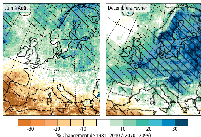
Fig. 74: Modifications des précipitations maximales de 5 jours sur l'Europe (en %) pour l'hiver et l'été vers 2070–2099, par rapport aux valeurs actuelles (1981–2010). La fig. montre les modifications de la médiane sur 15 modèles climatiques régionaux d'Euro-CORDEX avec une résolution d'env. 12 km. 147
