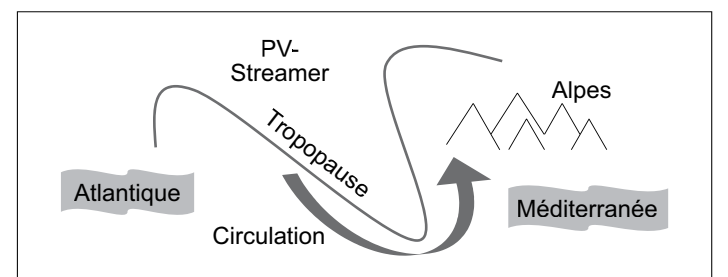
Fig. 7: Situation météo pendant l'inondation de septembre 1993. En haut : tropopause (trait tireté en gars), hauteur de l'isobare 200 hPa (lignes continues), soulèvement des masses d'air (zones grises, en Pa/s) et vent (flèches) dans la haute troposphère. En bas : représentation schématique de la situation. 20
