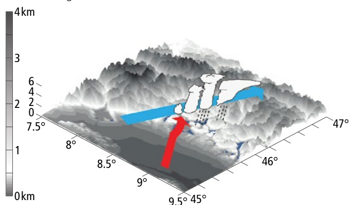
Fig. 14: Schéma conceptuel de la convection au-dessus de la région du lac Majeur. 34 L'air des basses couches en rouge, humide et conditionnellement instable, est forcé à monter lorsqu'il rencontre les Alpes. Des cellules convectives sont alors initiées, puis transportées par le flux des couches moyennes (en bleu). Les cellules convectives suivent des trajectoires similaires et produisent des précipitations au même endroit. Cette succession de cellules résulte localement en une forte accumulation de précipitation.
