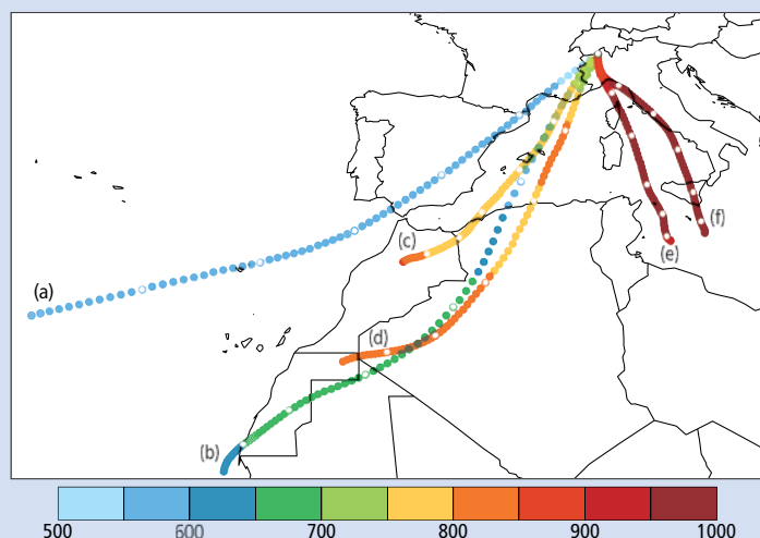
Fig. 12 : Trajectoires de parcelles d'air sur une période de 3 jours dans la réanalyse 20CR (cf p. 24). Les trajectoires se terminent à l'endroit 46°E 8°N le 27 septembre 1868 à 12 UTC pour les lignes (a), (c) et (e) et le 3 octobre 1868 à 12 UTC pour les lignes (b), (d) et (f). Les trajectoires se terminent à différentes altitudes, à savoir environ 5.5 km d'altitude (correspondant à 500 hPa) pour les lignes (a) et (b), 3 km (700 hPa) pour les lignes (c) et (d) et 1.5 km (850 hPa) pour les lignes (e) et (f). Les couleurs montrent la pression en hPa le long des trajectoires. Une pression haute indique qu'une parcelle d'air est proche du sol, une pression plus basse indique que cette parcelle se trouve à une altitude plus élevée. Un point blanc est ajouté chaque 12 heures. 32
