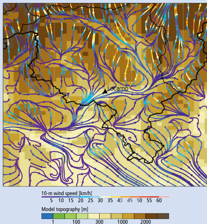
Fig. 46: Vent à 10m du sol le dimanche 27 septembre 1868 à 12h tel que reconstruit par le modèle WRF sur une grille de 2 km. La topographie du modèle est montrée en couleur, le vent par des flèches. La couleur des flèches représente la vitesse du vent. 32
