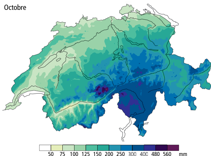
Fig. 31: Valeur mensuelle des précipitations en septembre et octobre 1868. 47
